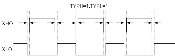
图 8.4a TYPH=1, TYPL=1 时的 PWM 波形输出
